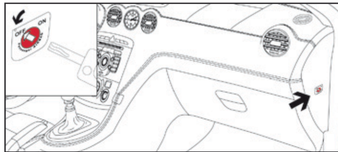
Отключение подушки безопасности пассажира ("OFF")
