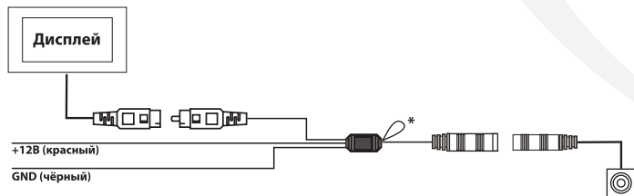
СХЕМА 1. Подключение камеры в качестве камеры переднего обзора (* необходимо обрезать белый провод)
