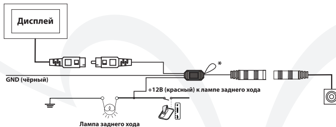
СХЕМА 2. Подключение камеры в качестве камеры заднего обзора (* не обрезать белый провод)
