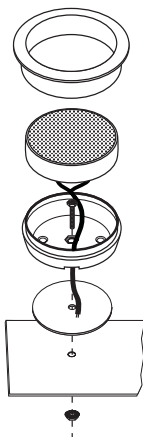
Вариант 3. Монтаж на поверхности.
