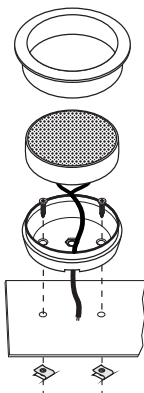
Вариант 4. Монтаж на поверхности.
