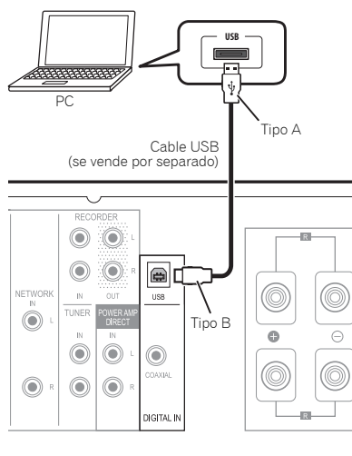
Panel posterior de la unidad A-70
