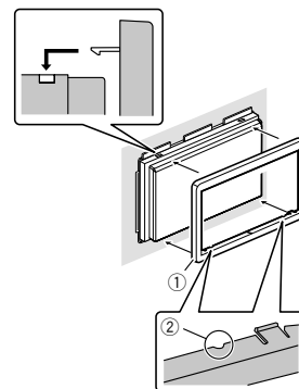
① Накладная рамка ② Паз
