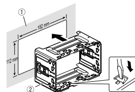
① Приборная панель ② Держатель
