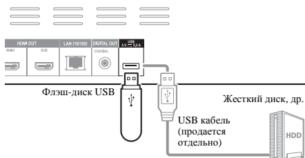
Задняя панель BDP-450
