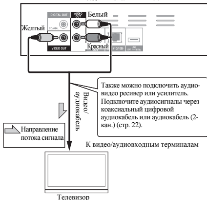
Задняя панель BDP-150
