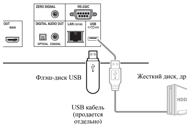
Задняя панель BDP-LX88
