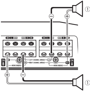
① Salida del altavoz (monoaural)
