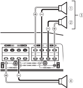
① Izquierda ② Derecha ③ Salida de altavoz A ④ Salida de altavoz B (monoaural) ■
