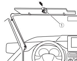
1 Microfoonklem
