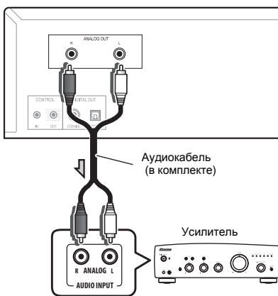
Задняя панель PD-30
