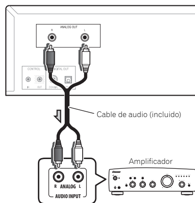
Panel posterior de la unidad PD-30
