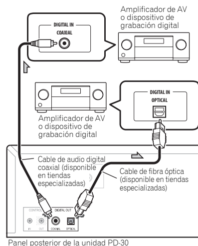
Panel posterior de la unidad PD-30
