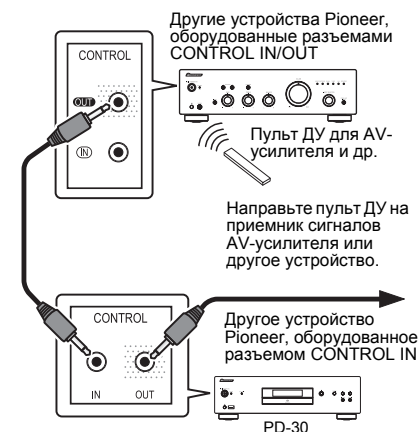
Задняя панель PD-30
