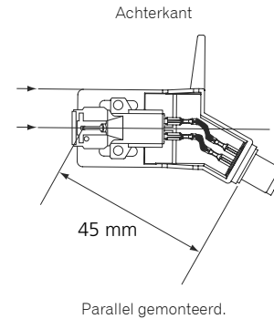
Parallel gemonteerd.
