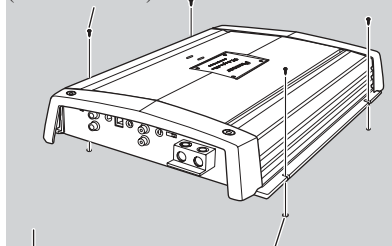
Blechschraube (4 mm × 18 mm)
