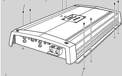
Zelftappende schroef (4 mm × 18 mm)
