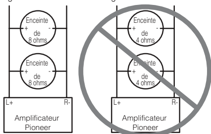
Branchement en pont de 4 ohms
