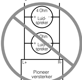
2 Ohm brugschakeling
