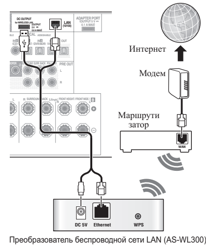
Преобразователь беспроводной сети LAN (AS-WL300)
