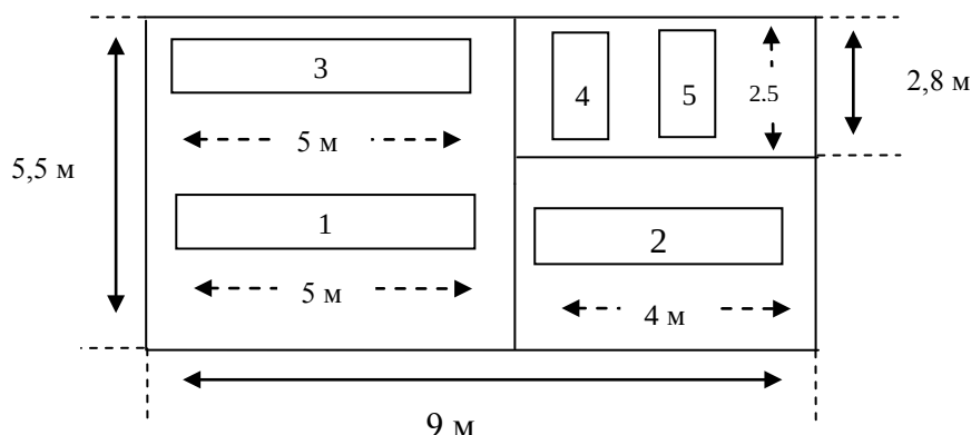
Рис. 5. План помещения
