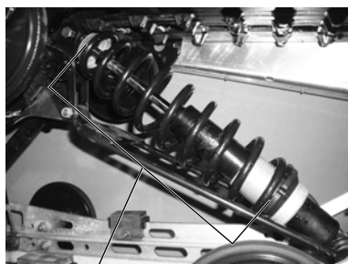
Длина пружины
