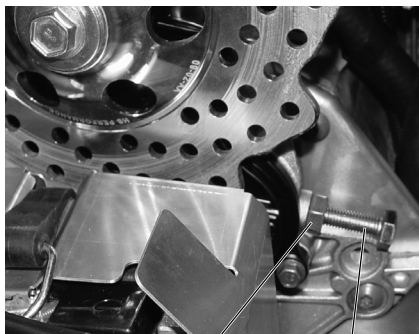
Контргайка. Регулировочный болт
