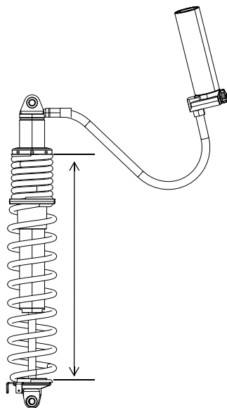
Измерение предварительной затяжки заднего амортизатора
