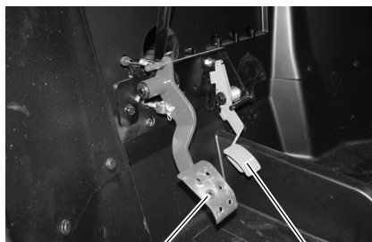
Педаль газа
