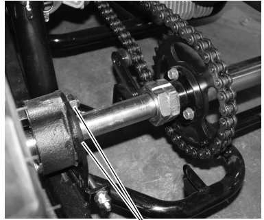
Болты крепления задней оси
