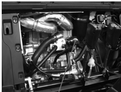
Масляный фильтр
