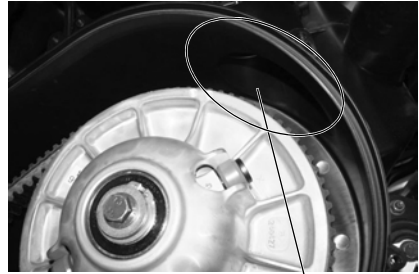
Воздуховоды вариатора
