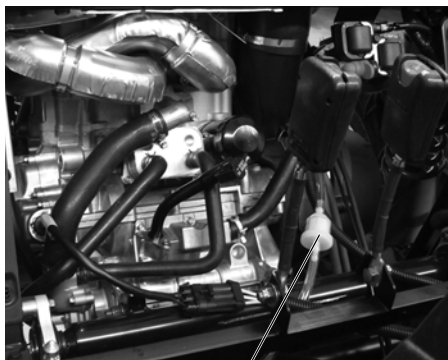
Фильтр вентиляции бензобака
