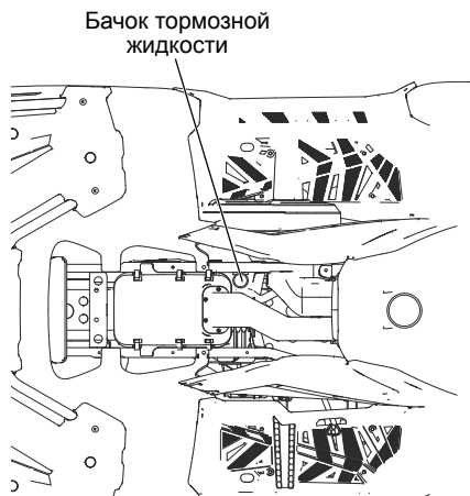
Дополнительный ножной тормоз
