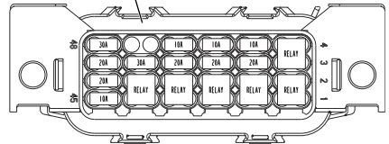
Блок предохранителей
