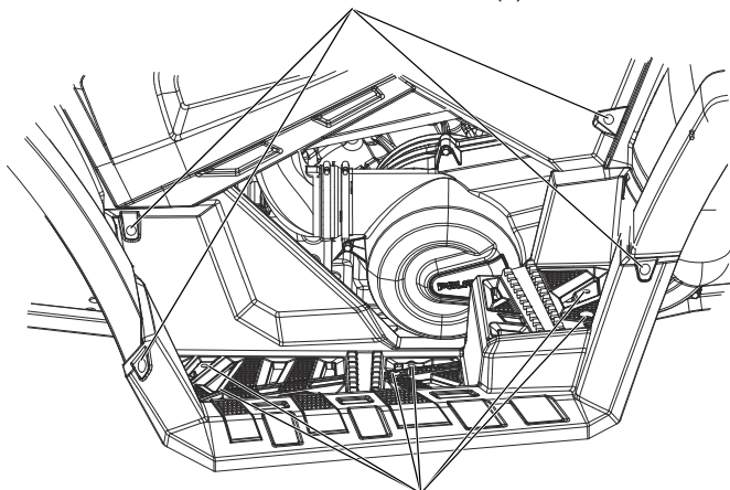
Винты Torx (6)
