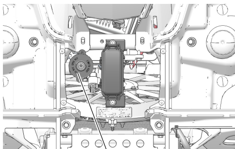
Крышка радиатора
