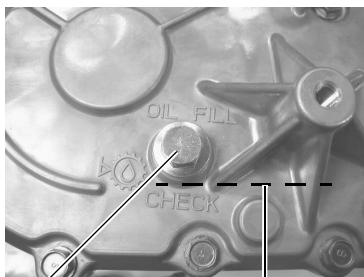
Заливная пробка
