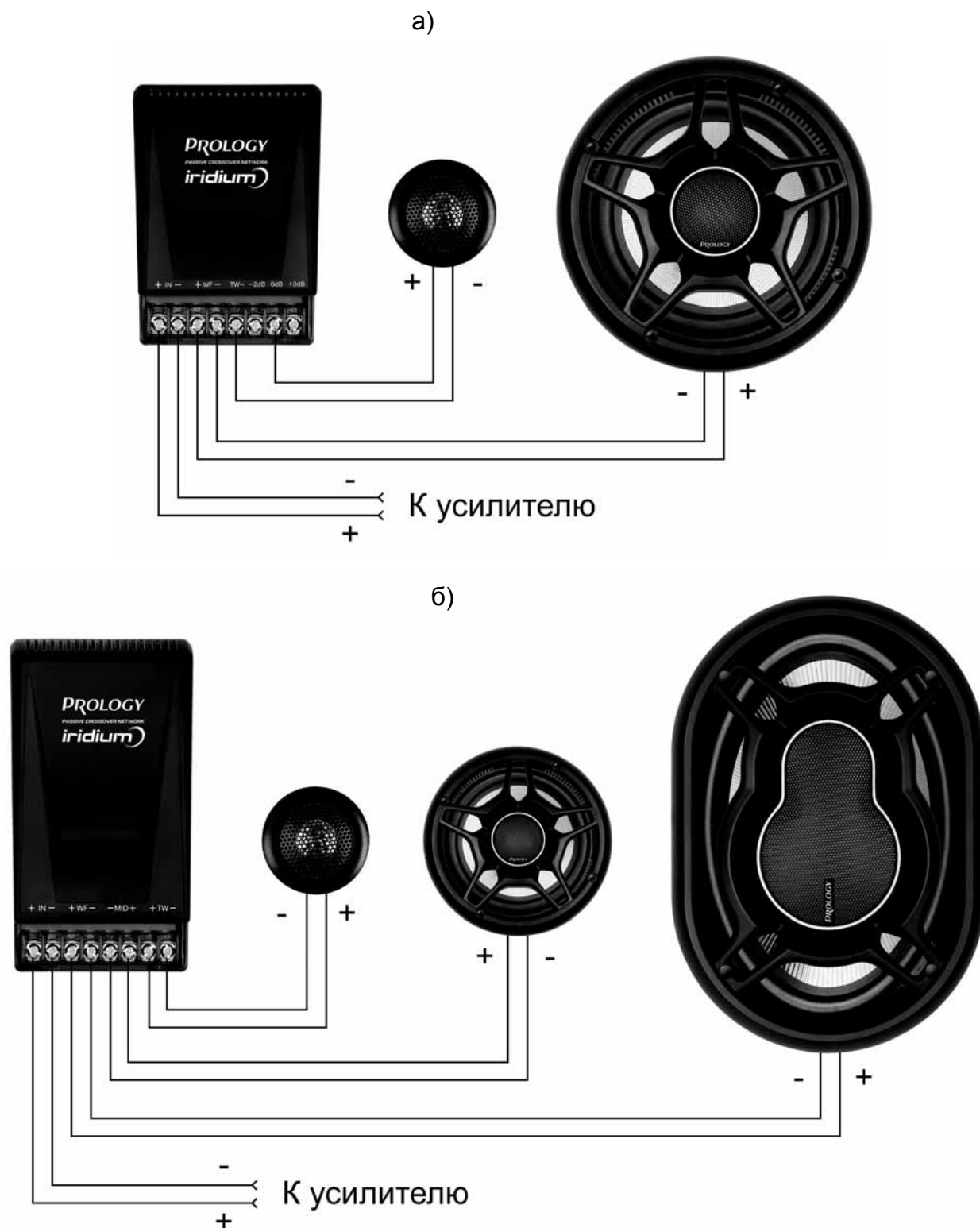
Рис. 3. Схема подключения 2-полосной (а) и 3-полосной (б) акустической системы
