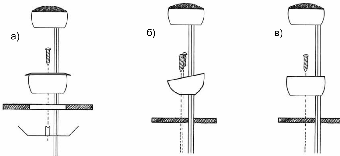
Схема установки ВЧ-динамика
