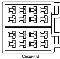
Расположение контактов разъема ISO:
