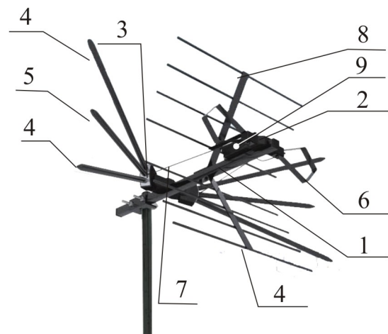
Рис.1 Внешний вид антенны «Колибри- А-DX De Luxe»
