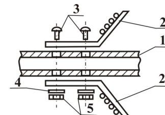
Рис.2 Схема сборки и установки комплекта рефлекторов «DeLuxe»
