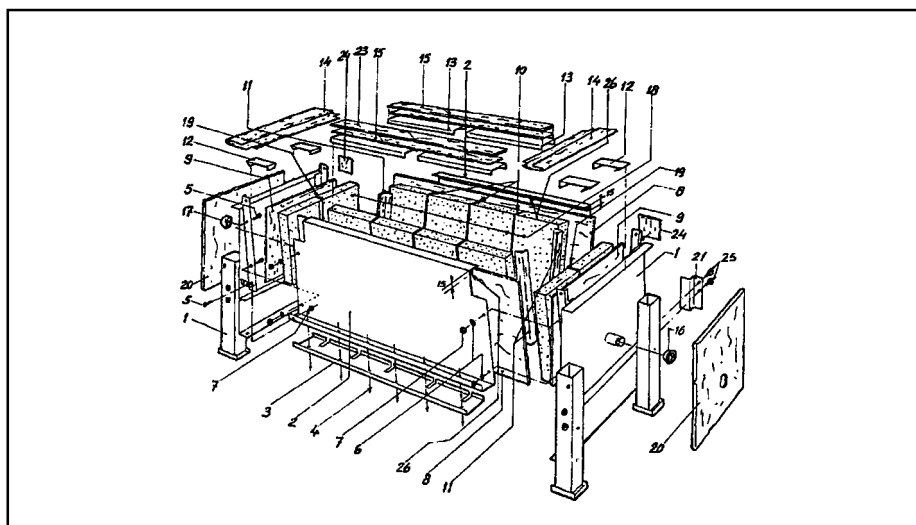
Рис. 5. Топочная камера
