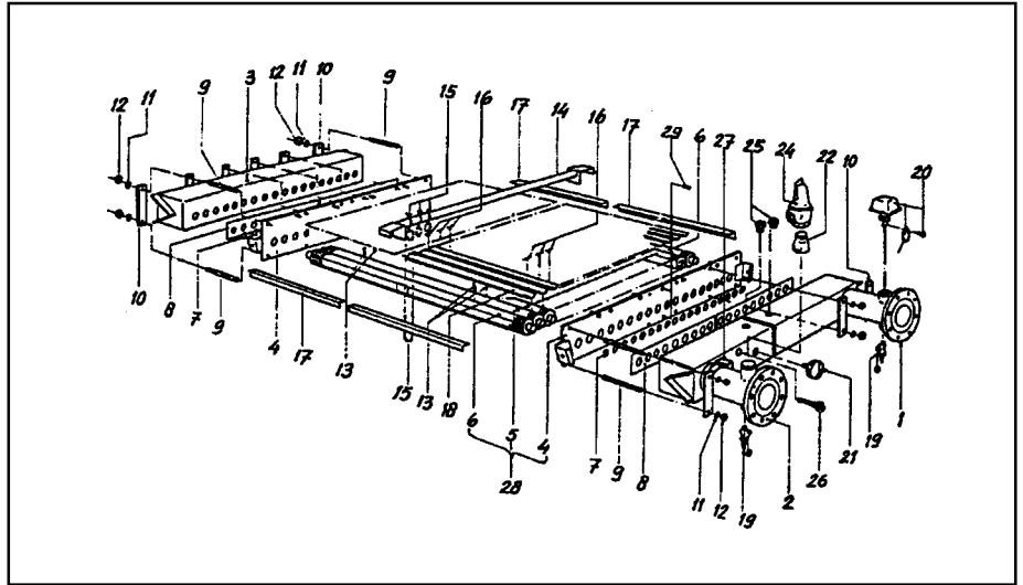
Рис. 6. Теплообменник
