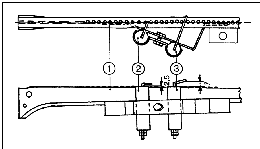
Рис. 32. Электроды
