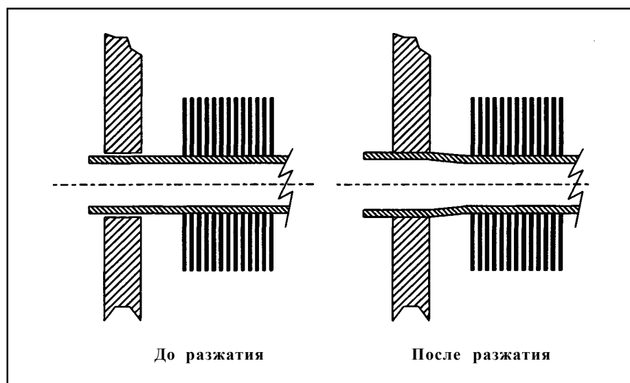
Рис. 35. Разжатие концов оребренных трубок
