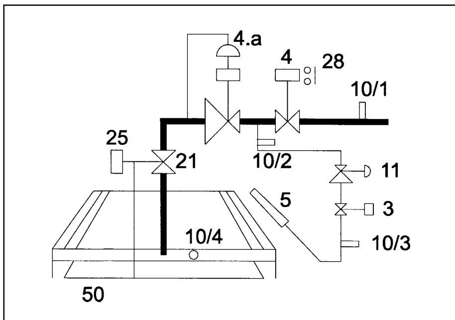
Рис. 33. Газовая схема
