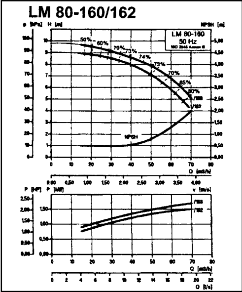
Рис. 26. Характеристики насоса LM 80-160/162
