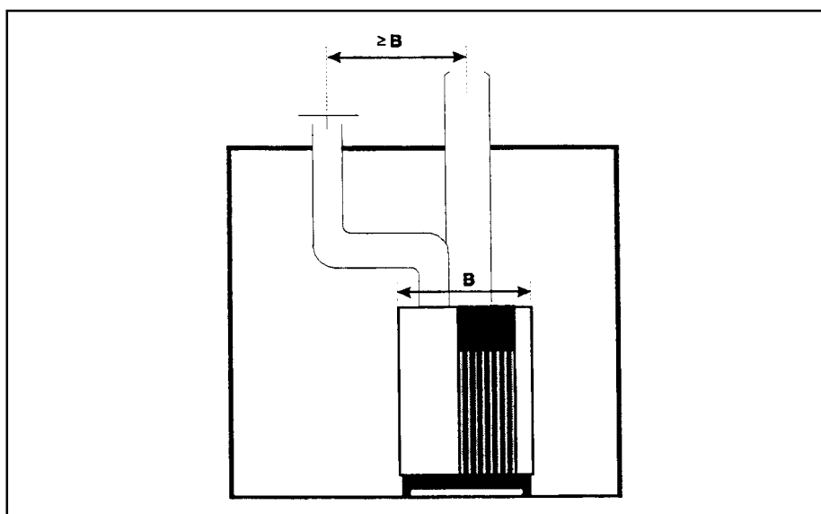
Рис. 21. Расстояние между входом воздуховода и выходом дымохода
