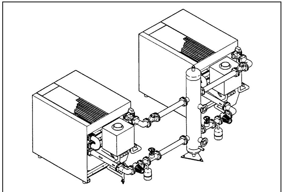
Рис. 31. Водосборник низкой скорости для двух котлов
