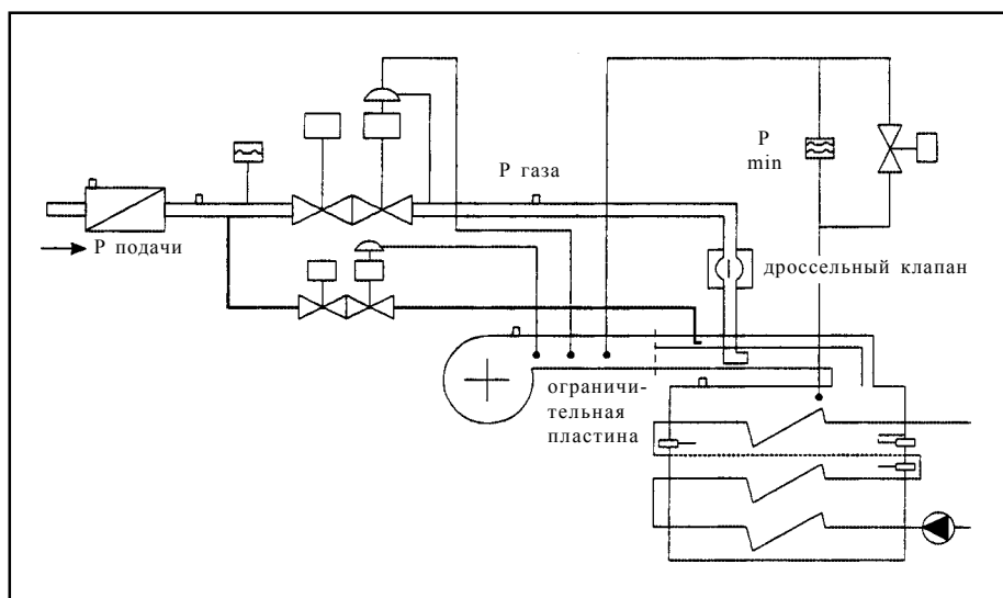
Рис. 33. Измерение давления в горелке
