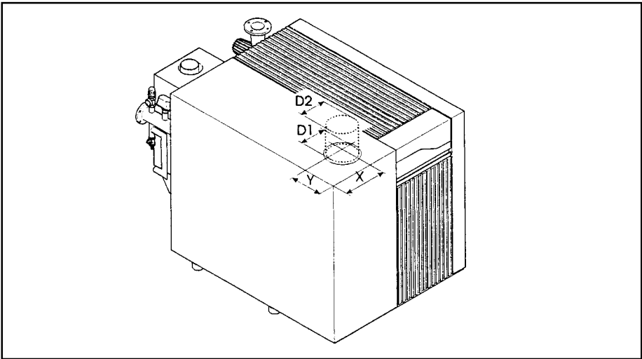
Рис. 19. Присоединение воздуховода
