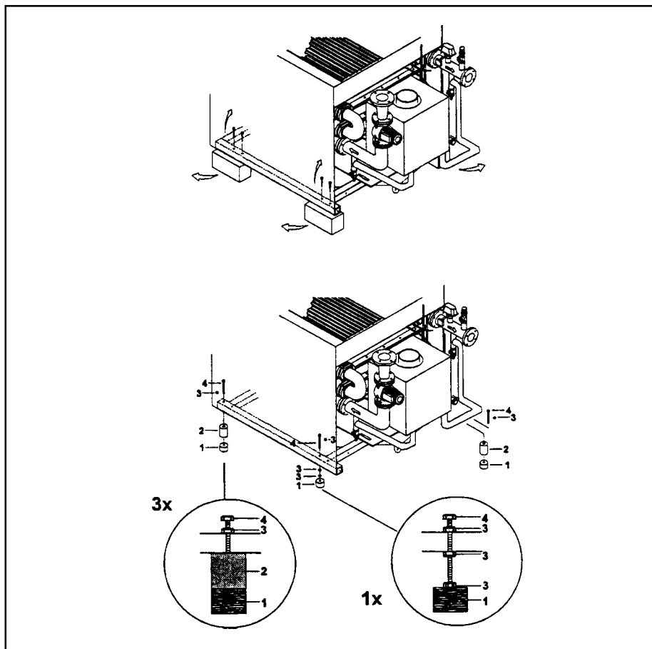
Рис. 13. Монтаж амортизаторов
