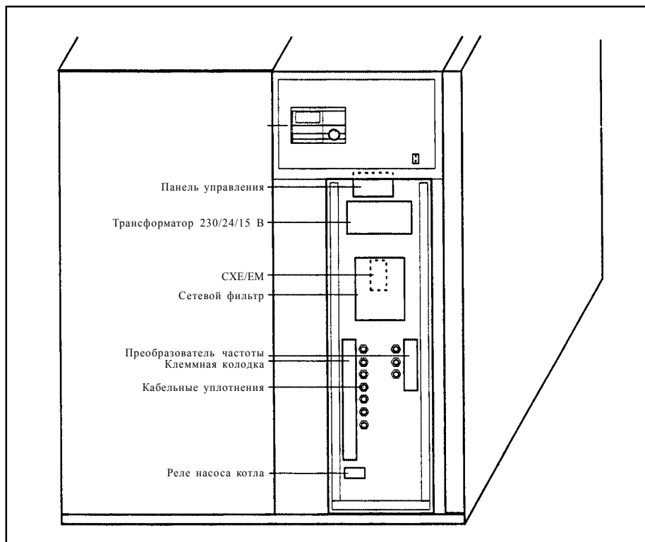
Рис. 16. Соединительная коробка
