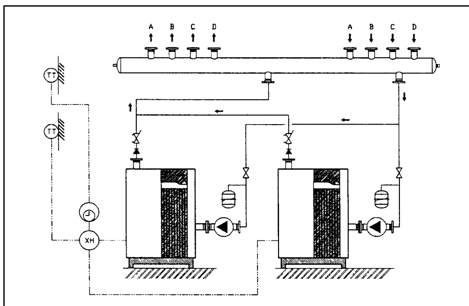
Рис. 29. Установка с несколькими котлами
