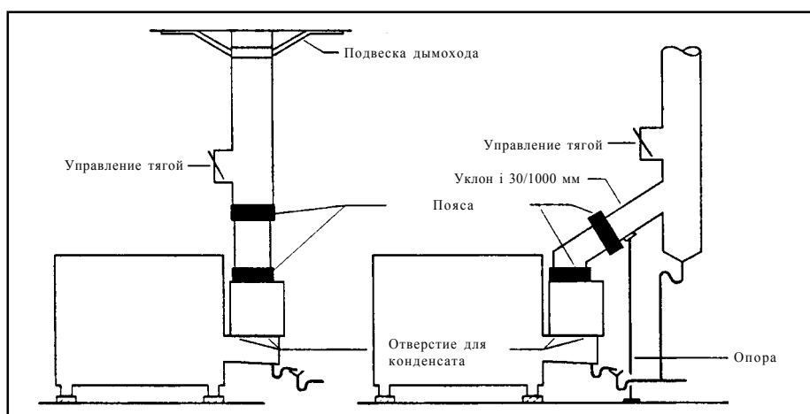
Рис. 22б. Присоединение дымохода в R3600
