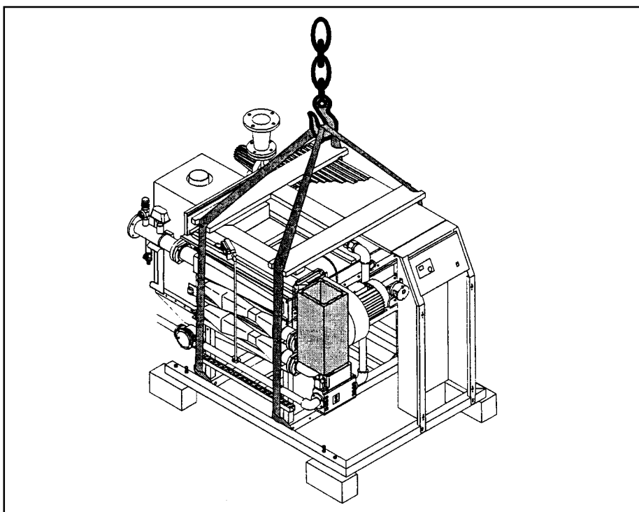
Рис. 8. Подъем
