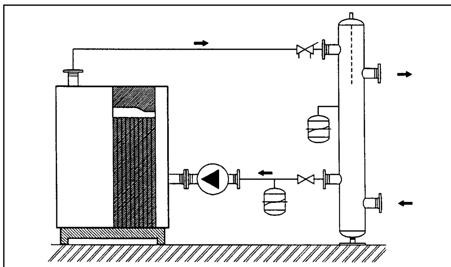
Рис. 27. Установка с водосборником низкой скорости, запорным клапаном и расширительным баком
