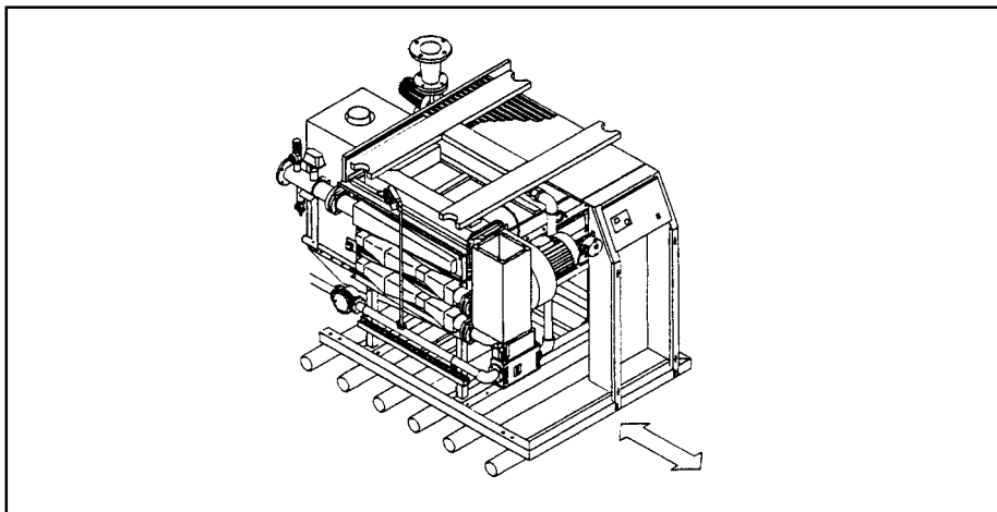
Рис. 7. Перемещение установки с помощью катков.
