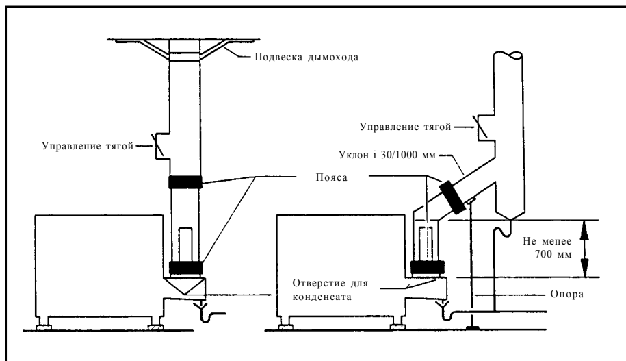
Рис. 22а. Присоединение дымохода в R3400/R3500
