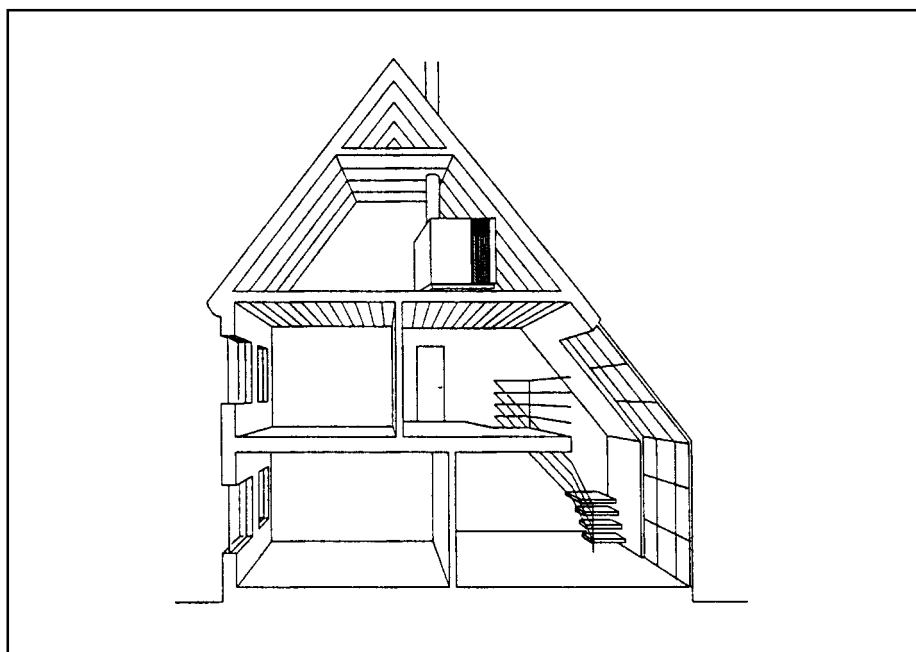
Рис. 15. Установка на чердаке
