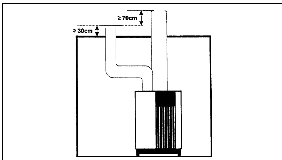
Рис. 20. Высоты входа воздуховода и выхода дымохода
