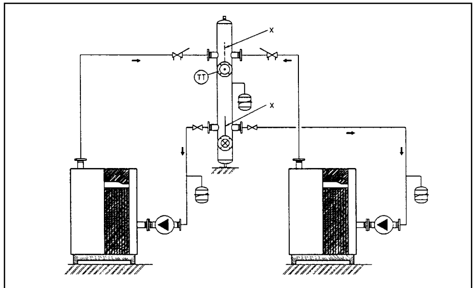
Рис. 30. Установка с несколькими котлами без обратных клапанов и использованием водосборника низкой скорости для двух котлов
