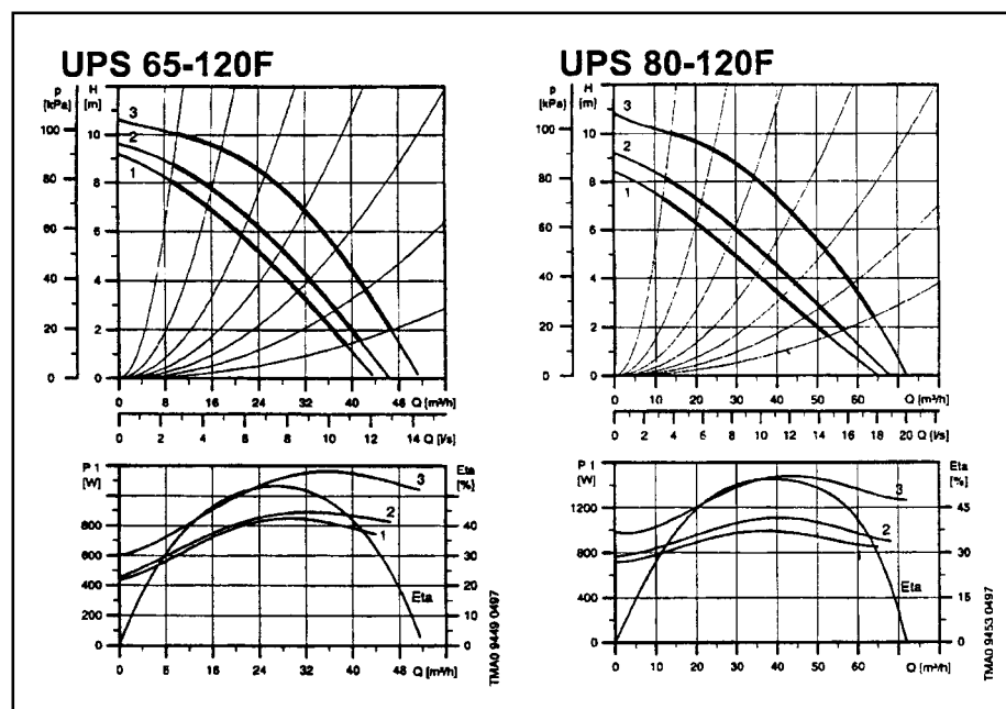
Рис. 24. Характеристики насоса UPS 65-120F
