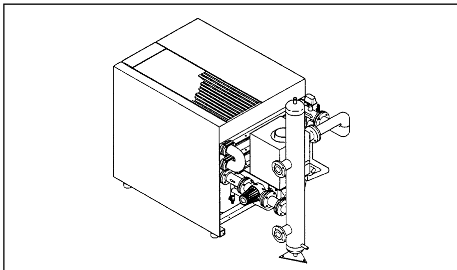
Рис. 28. Котел с установленным вертикально водосборником низкой скорости с правосторонними подключениями
