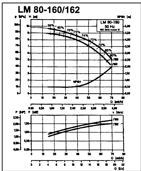
Рис. 26. Характеристики насоса LM 80-160/162
