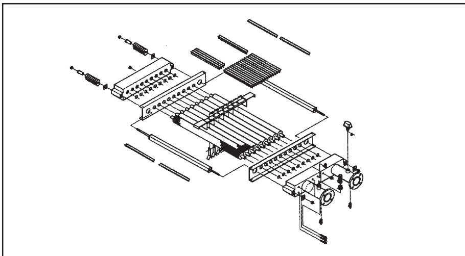
Рис. 5. Теплообменник
