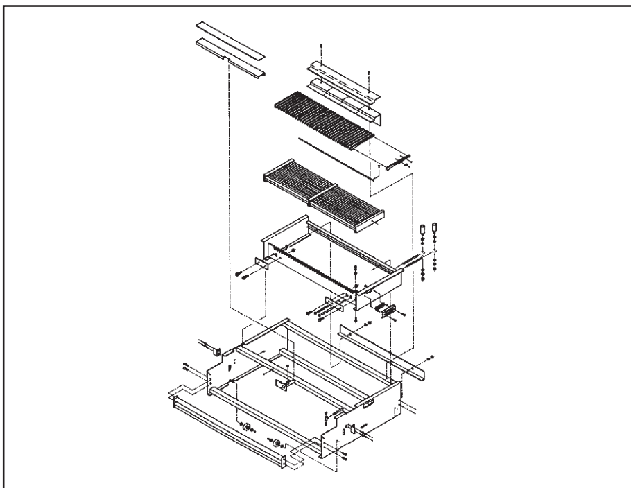
Рис. 6. Горелка
