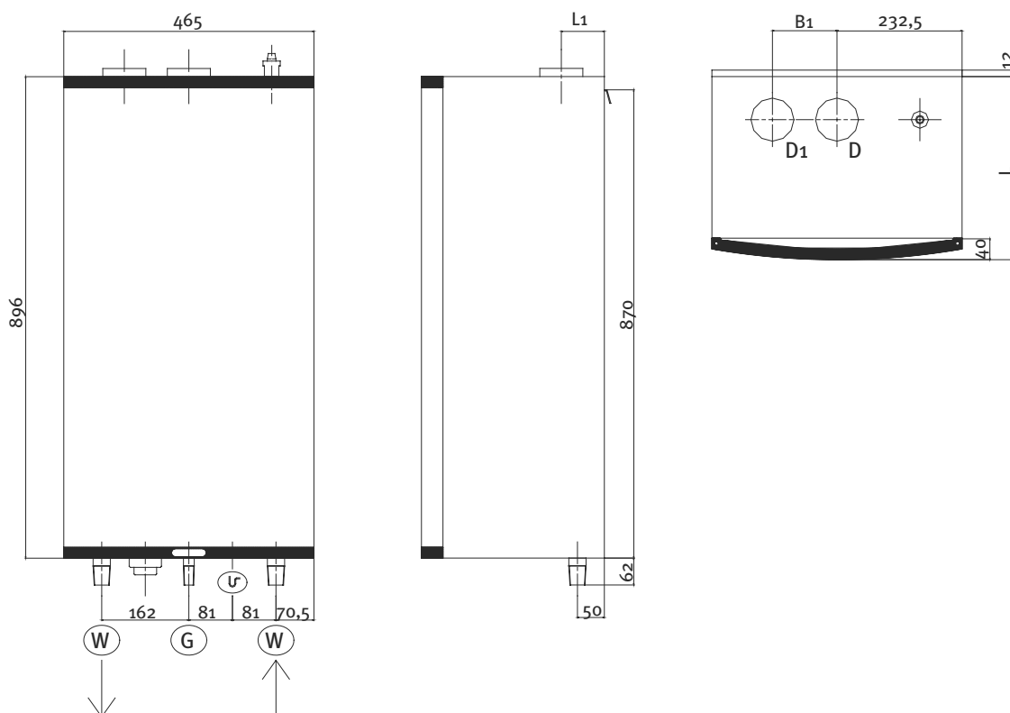
Рис. 1 Размеры R30
