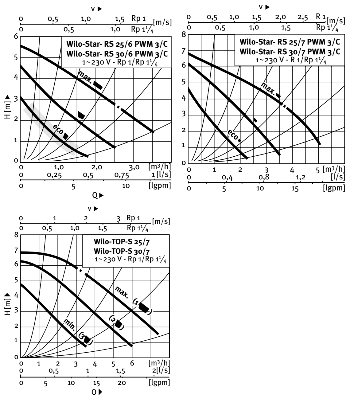
Рис. 5 Характеристика насоса
