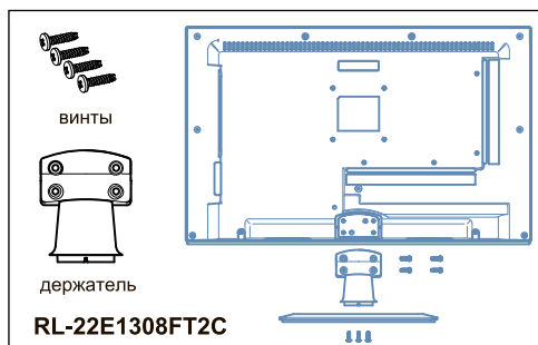
ВИНТЫ
