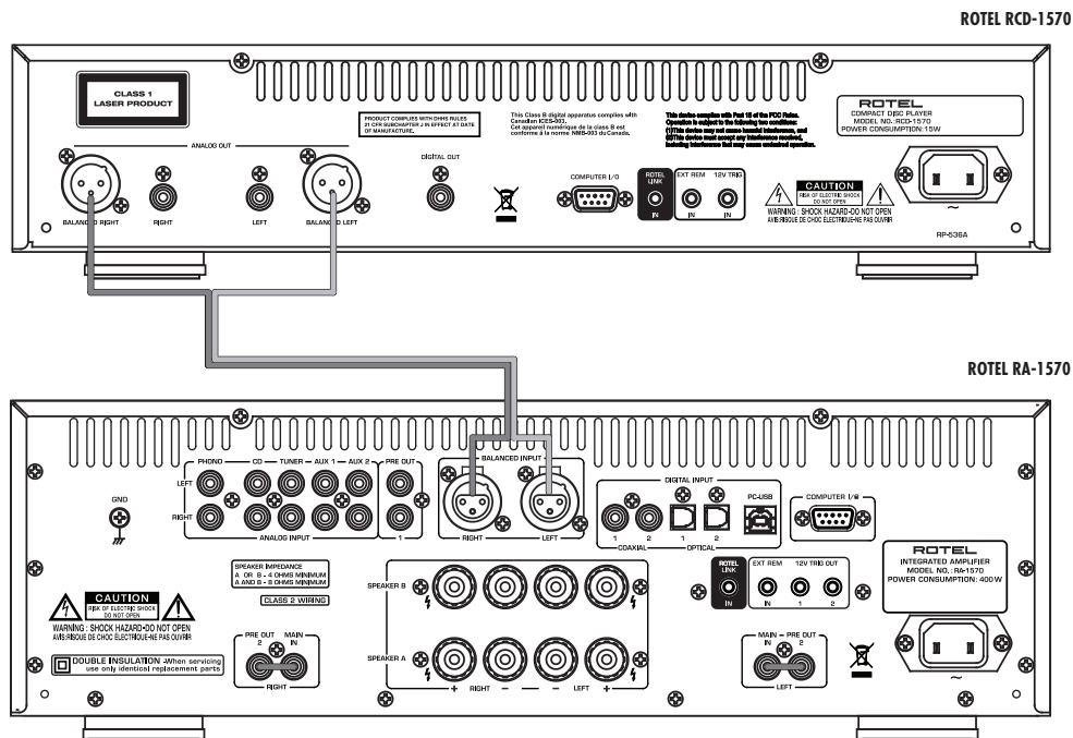
Figure 4: Balanced Outputs Sorties symétriques Symmetrische Ausgänge Salidas Balanceadas
