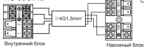
RS-09UIN1
