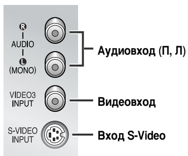
Боковая панель телевизора
