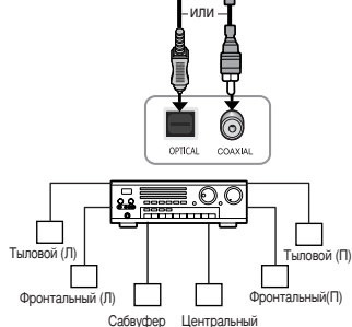
К цифровому аудиовыходу AV-ресивера с декодером Dolby Digital, MPEG2 или DTS
