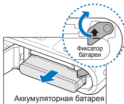
Аккумуляторная батарея
