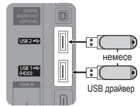
Теледидардың артқы панелі
