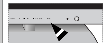
Передняя панель ПД
