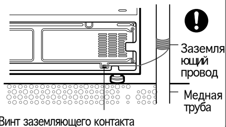
Винт заземляющего контакта
