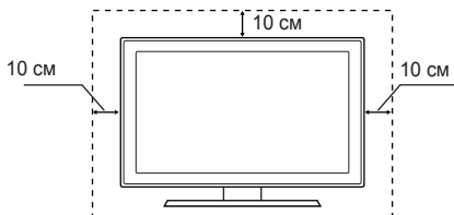
Тұрғыға орнату
