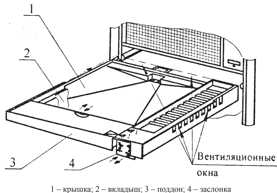
Рисунок 2 – Схема установки поддона
