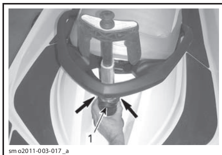
ТИПОВОЙ ВАРИАНТ — ЧТОБЫ ОСВОБОДИТЬ И ОПУСТИТЬ ПИЛОН, НАЖМИТЕ В НАПРАВЛЕНИИ НОСОВОЙ ЧАСТИ
