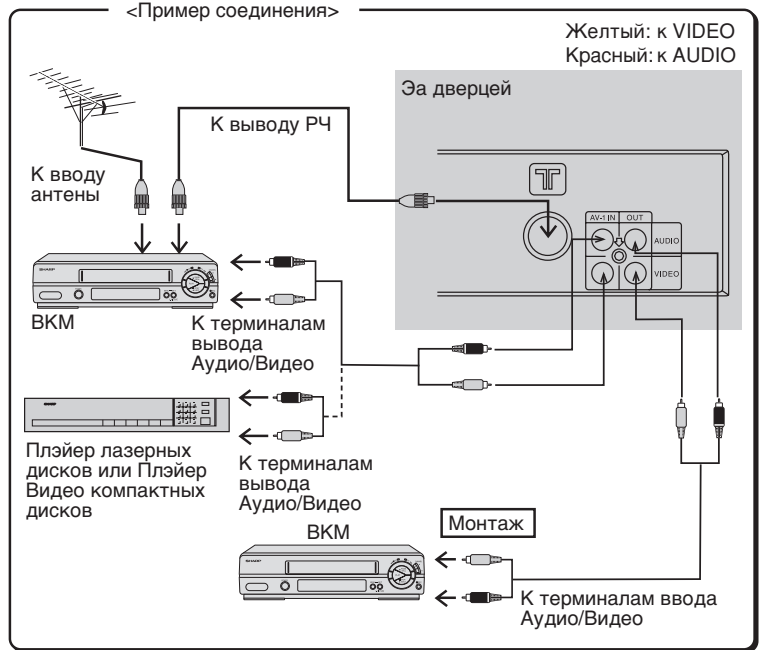
<Пример соединения>
