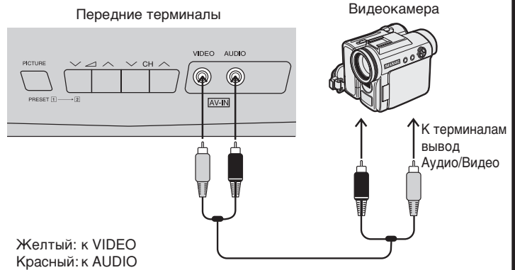
<Пример соединения>
