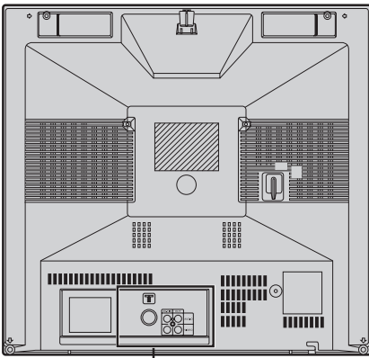
ЗАДНЯЯ ПАНЕЛЬ
