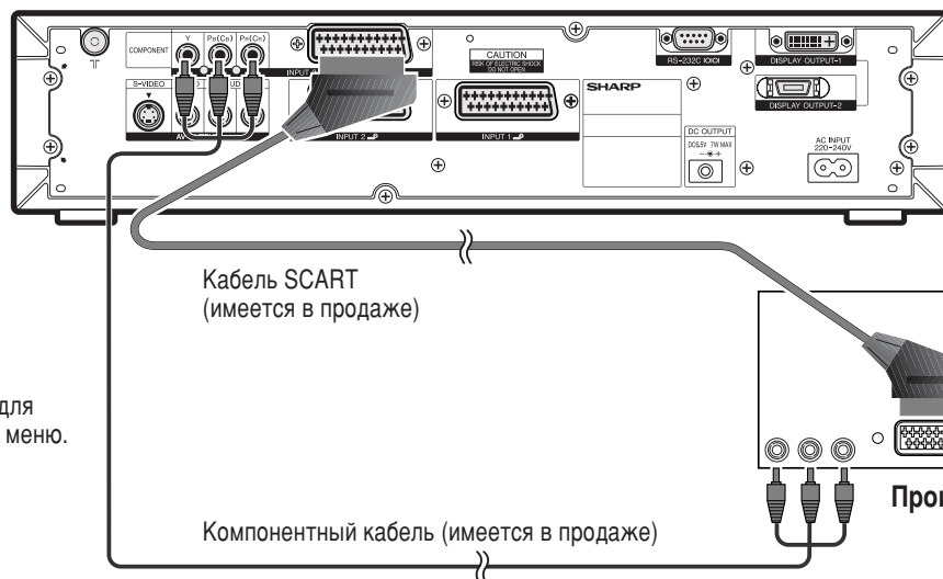
Система AVC (вид сзади)
