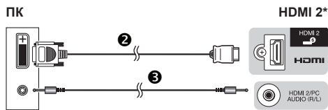
2 Кабель DVI/HDMI 3 Стерефонический кабель с минигнездом Ø 3,5 мм
