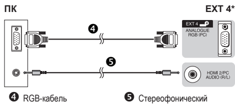
4 RGB-кабель 5 Стерефонический кабель с минигнездом Ø 3,5 мм
