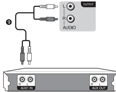
9 Аудиокабель
