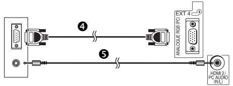
4 RGB-кабель 5 Стерефонический кабель с минигнездом Ø 3,5 мм
