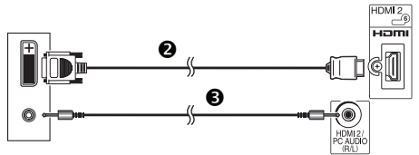
2 Кабель DVI/HDMI 3 Стерефонический кабель с минигнездом Ø 3,5 мм
