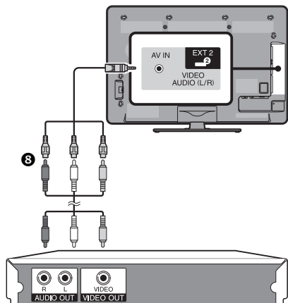
8 Кабель AV (входит в комплект)/Переходной кабель
